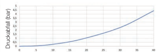
Druckabfall NSA ø8 Wasser
