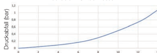
Druckabfall NSA ø6 Wasser
